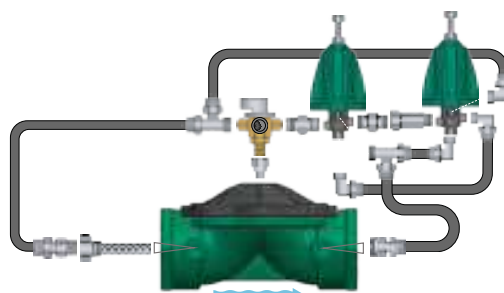
ELETTROVALVOLA REGOLATRICE DI PRESSIONE
