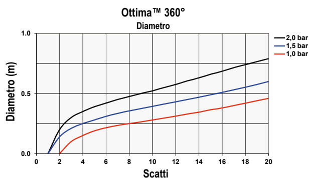
Ottima™ 360° Filetto 10-32 UNF
