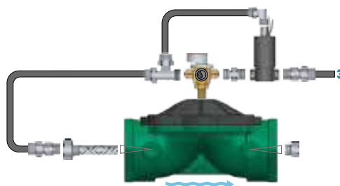
ELETTROVALVOLA CON COMANDO MANUALE (N.C)
