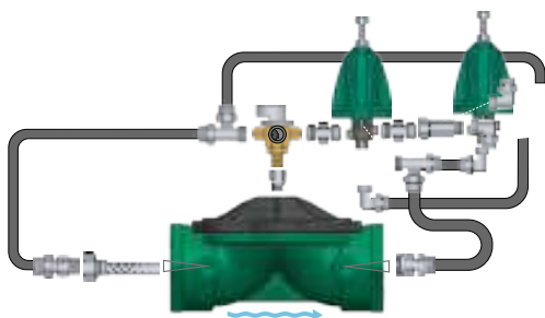
VALVOLA DI REGOLAZIONE E SOSTEGNO DI PRESSIONE
