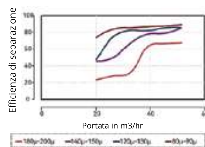
Diagramma della efficienza della separazione centrifuga per 4
