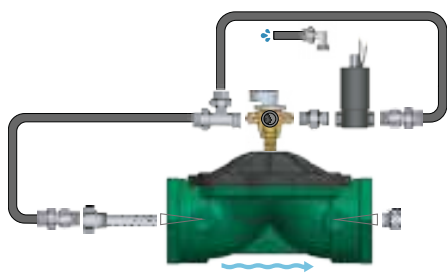
ELETTROVALVOLA CON COMANDO MANUALE (N.O)
