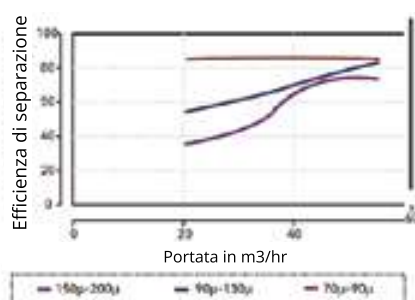
Diagramma della efficienza della separazione centrifuga per 3
